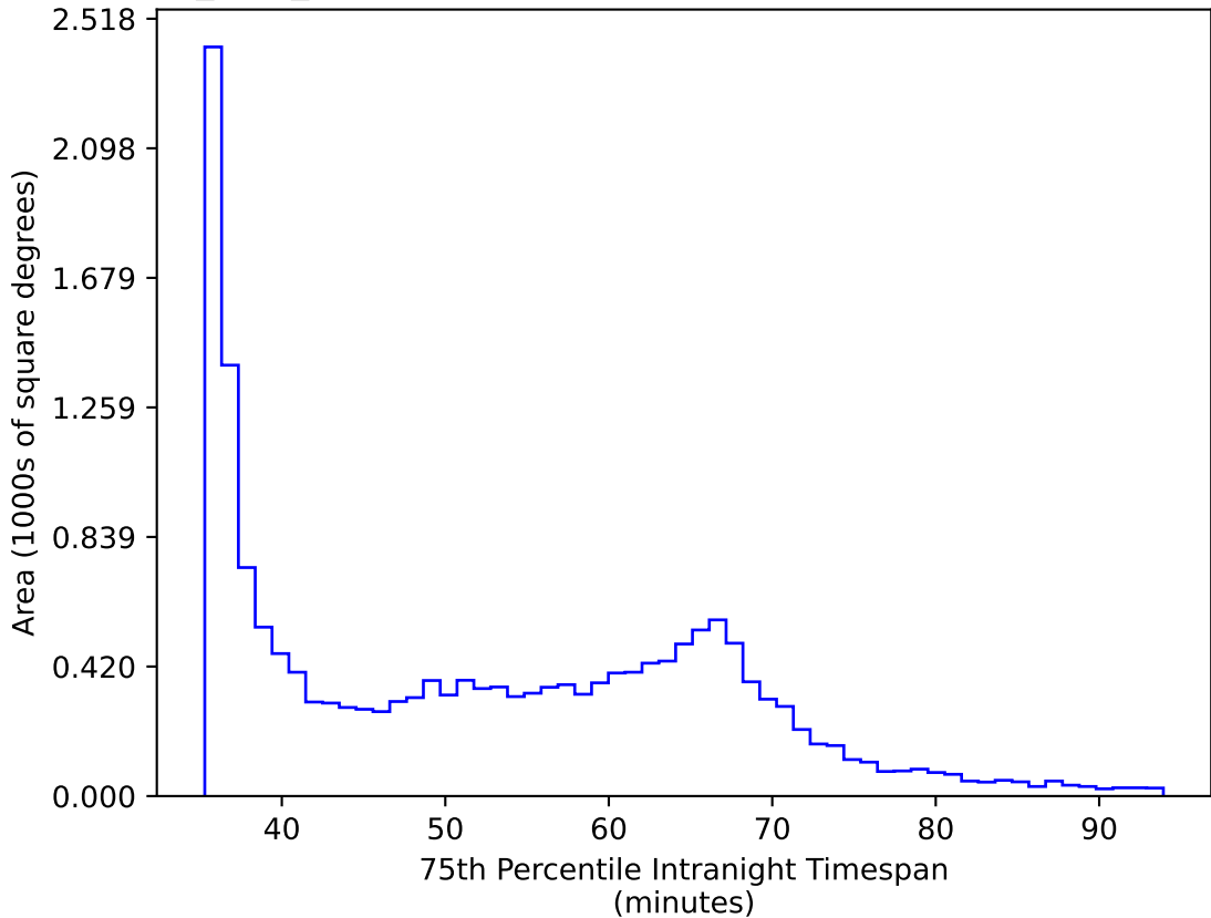
baseline_v2.0_10yrs WFD iz bands: 75th Percentile Intranight Timespan
