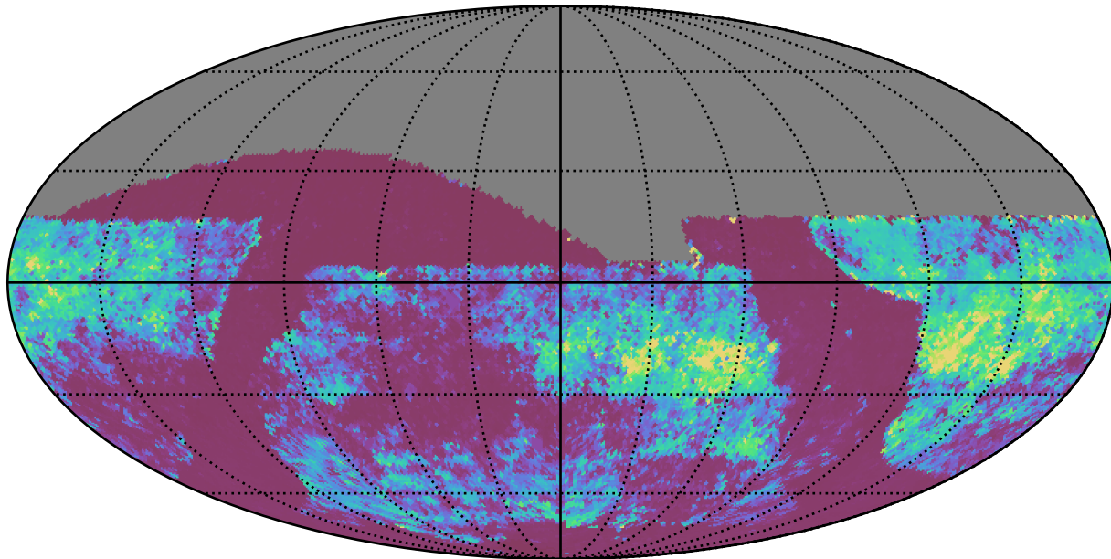
baseline_v2.0_10yrs All sky iz bands: 75th Percentile Intranight Timespan
