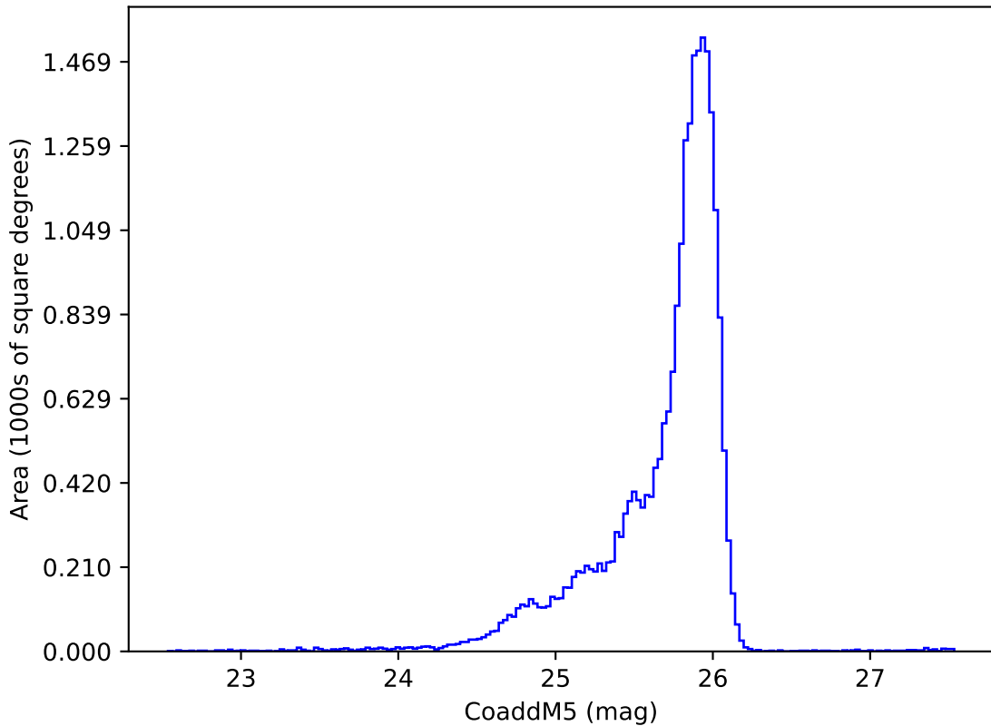
baseline_v2.0_10yrs u: CoaddM5
