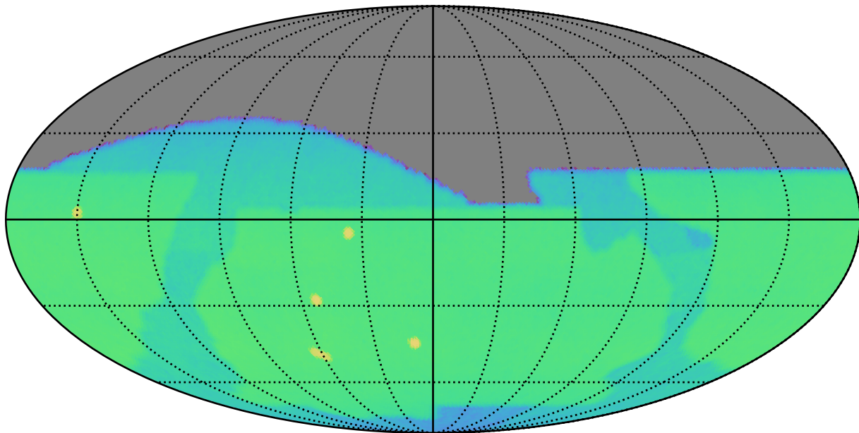
baseline_v2.0_10yrs i: CoaddM5
