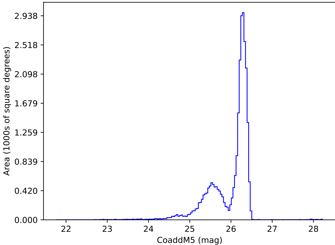
baseline_v2.0_10yrs i: CoaddM5
