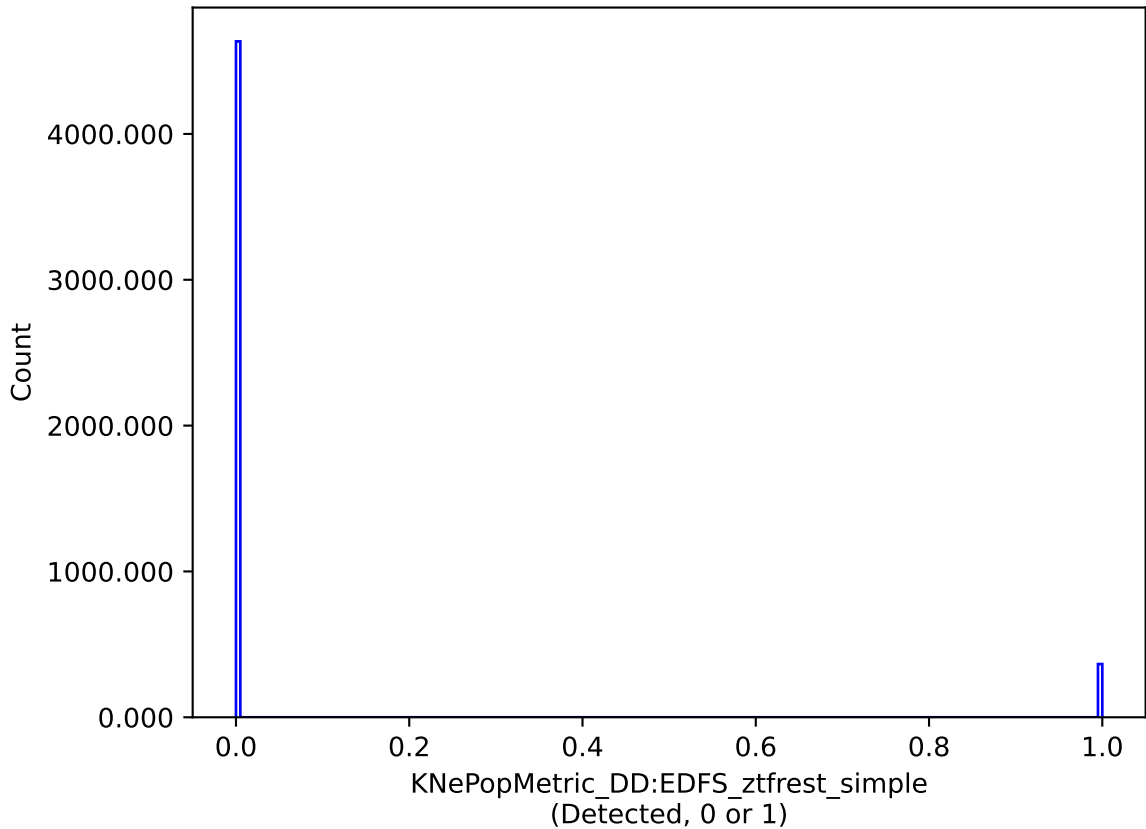
baseline_v2.0_10yrs DD:EDFS: KNePopMetric_DD:EDFS_ztfrest_simple
