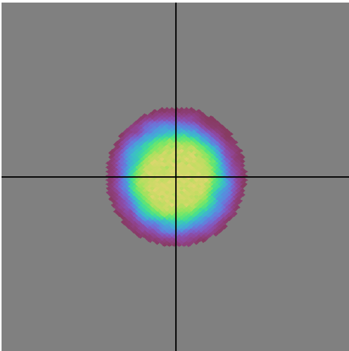
baseline_v2.0_10yrs z band: DD:XMM_LSS NVisits
