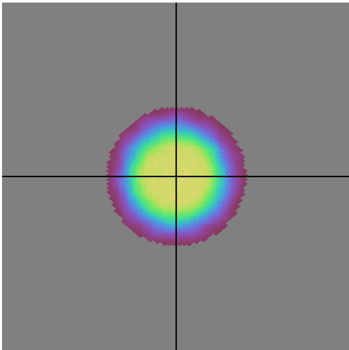
baseline_v2.0_10yrs r band: DD:XMM_LSS NVisits
