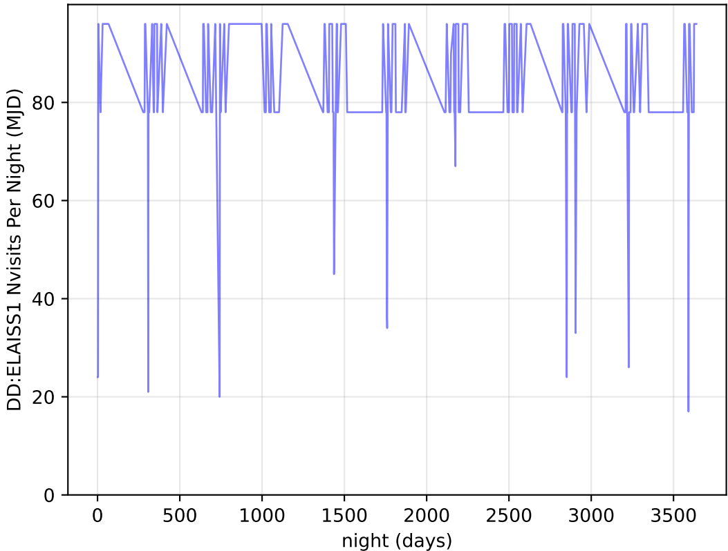
baseline_v2.0_10yrs all bands: DD:ELAISS1 Nvisits Per Night
