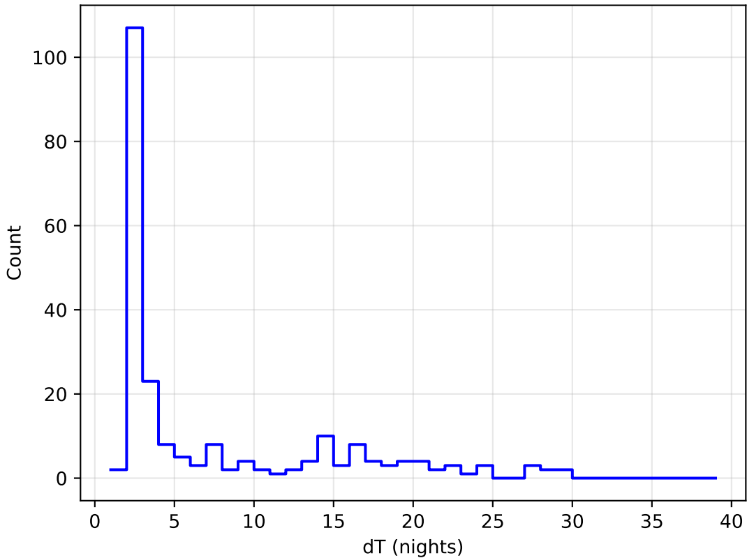
baseline_v2.0_10yrs all bands: DD:ELAISS1 Delta Nights Histogram
