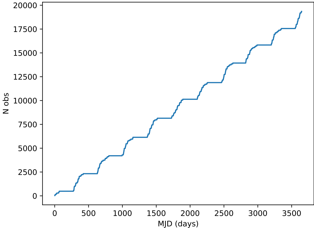
baseline_v2.0_10yrs all bands: DD:ELAISS1 Cumulative NVisits
