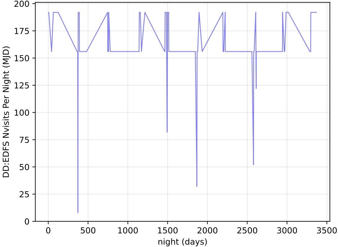
baseline_v2.0_10yrs all bands: DD:EDFS Nvisits Per Night
