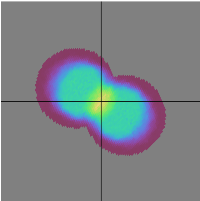
baseline_v2.0_10yrs u band: DD:EDFS NVisits
