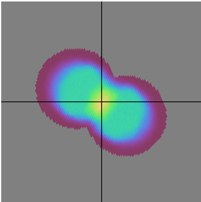
baseline_v2.0_10yrs r band: DD:EDFS NVisits
