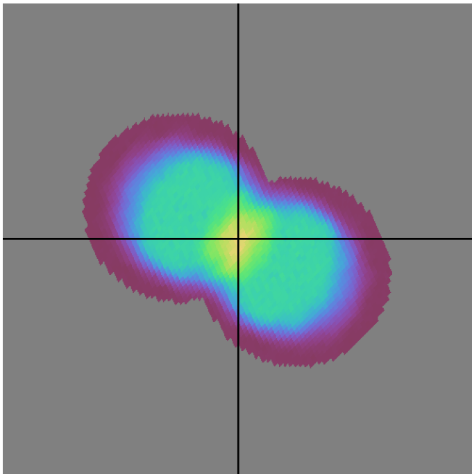
baseline_v2.0_10yrs g band: DD:EDFS NVisits
