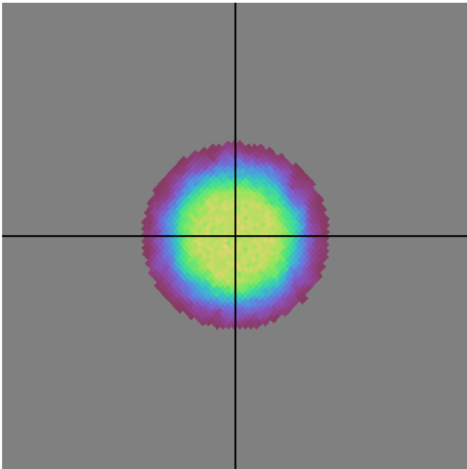
baseline_v2.0_10yrs z band: DD:ECDFS NVisits
