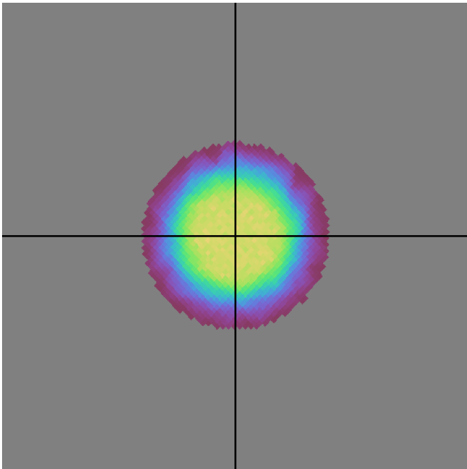
baseline_v2.0_10yrs y band: DD:ECDFS NVisits
