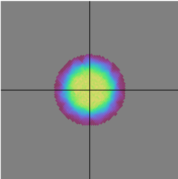
baseline_v2.0_10yrs u band: DD:ECDFS NVisits
