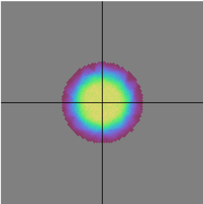
baseline_v2.0_10yrs r band: DD:ECDFS NVisits
