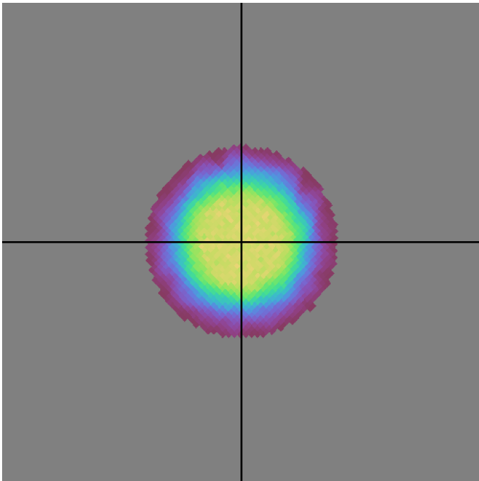
baseline_v2.0_10yrs g band: DD:ECDFS NVisits
