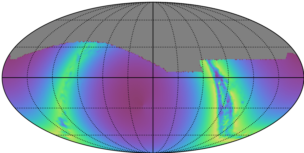
all_long_v3.4_10yrs : young_stars
