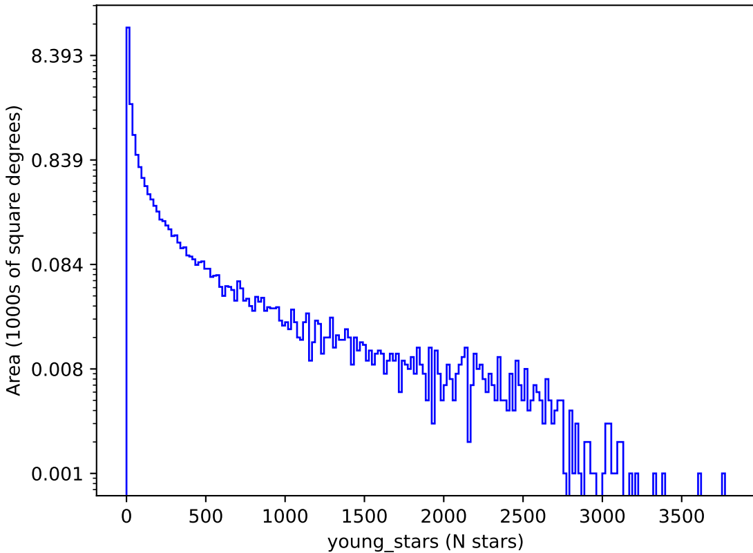
all_long_v3.4_10yrs : young_stars
