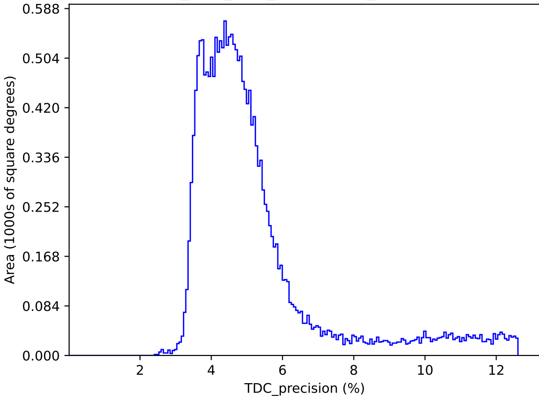
all_long_v3.4_10yrs : TDC_precision
