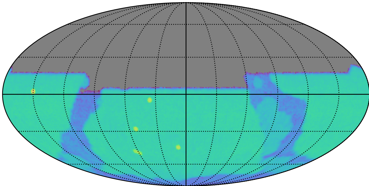
all_long_v3.4_10yrs u: SurfaceBrightLimit
