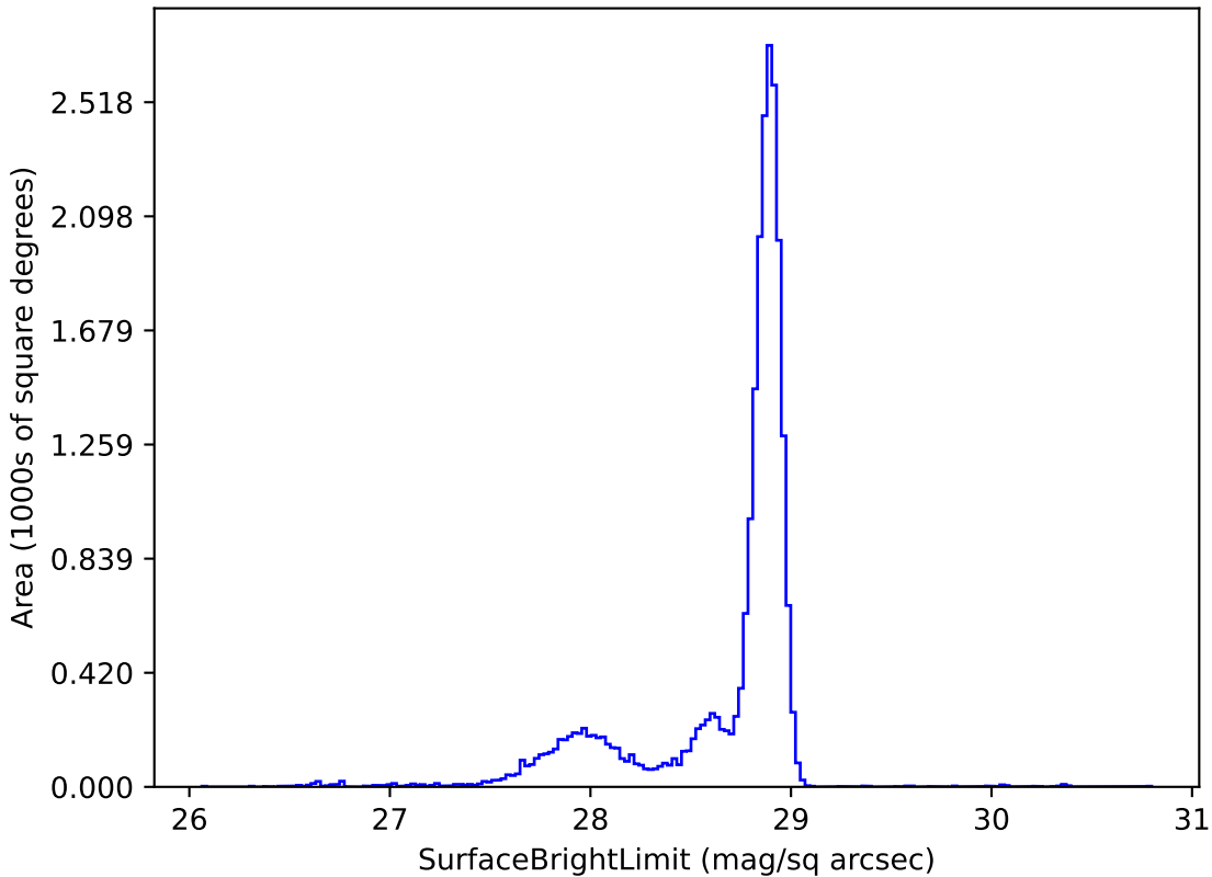
all_long_v3.4_10yrs u: SurfaceBrightLimit
