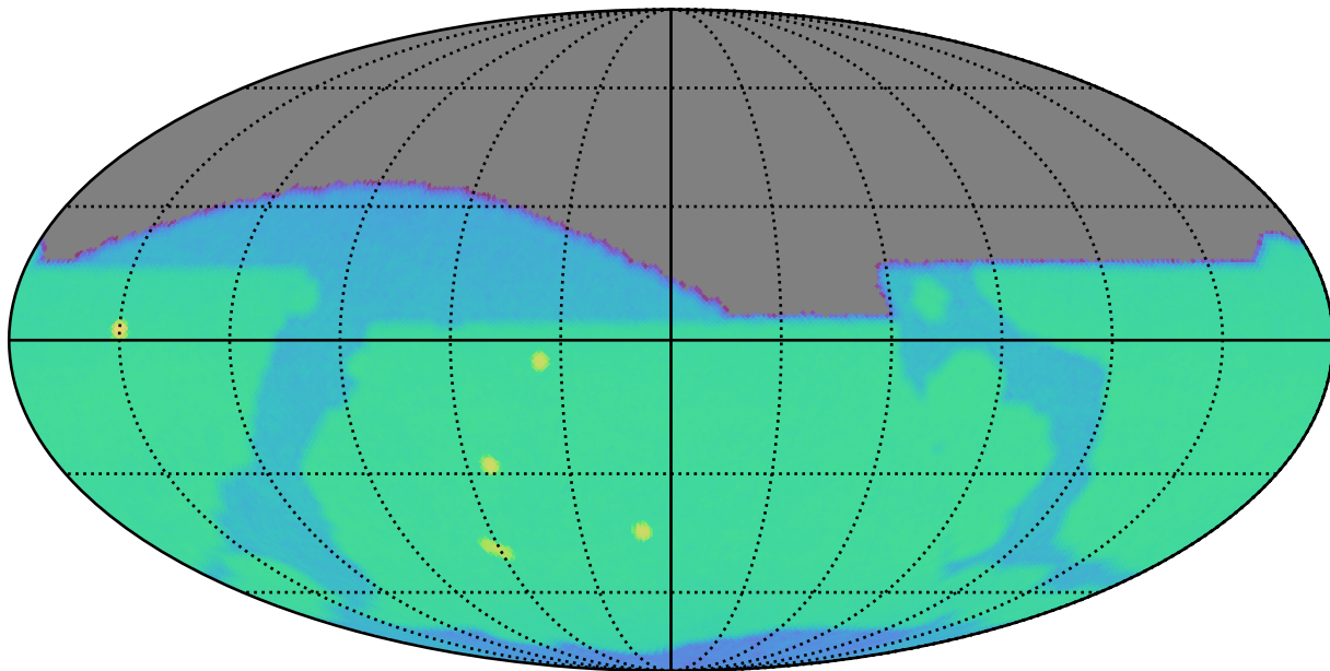
all_long_v3.4_10yrs i: SurfaceBrightLimit
