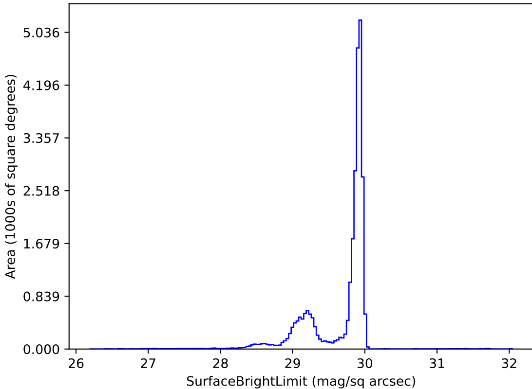
all_long_v3.4_10yrs i: SurfaceBrightLimit
