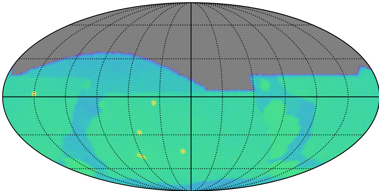
all_long_v3.4_10yrs g: SurfaceBrightLimit
