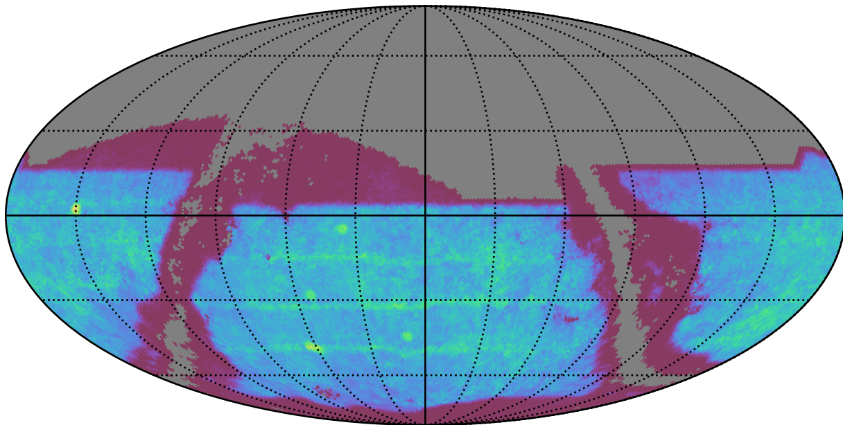
all_long_v3.4_10yrs : SNSLMetric
