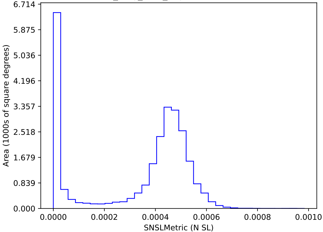
all_long_v3.4_10yrs : SNSLMetric
