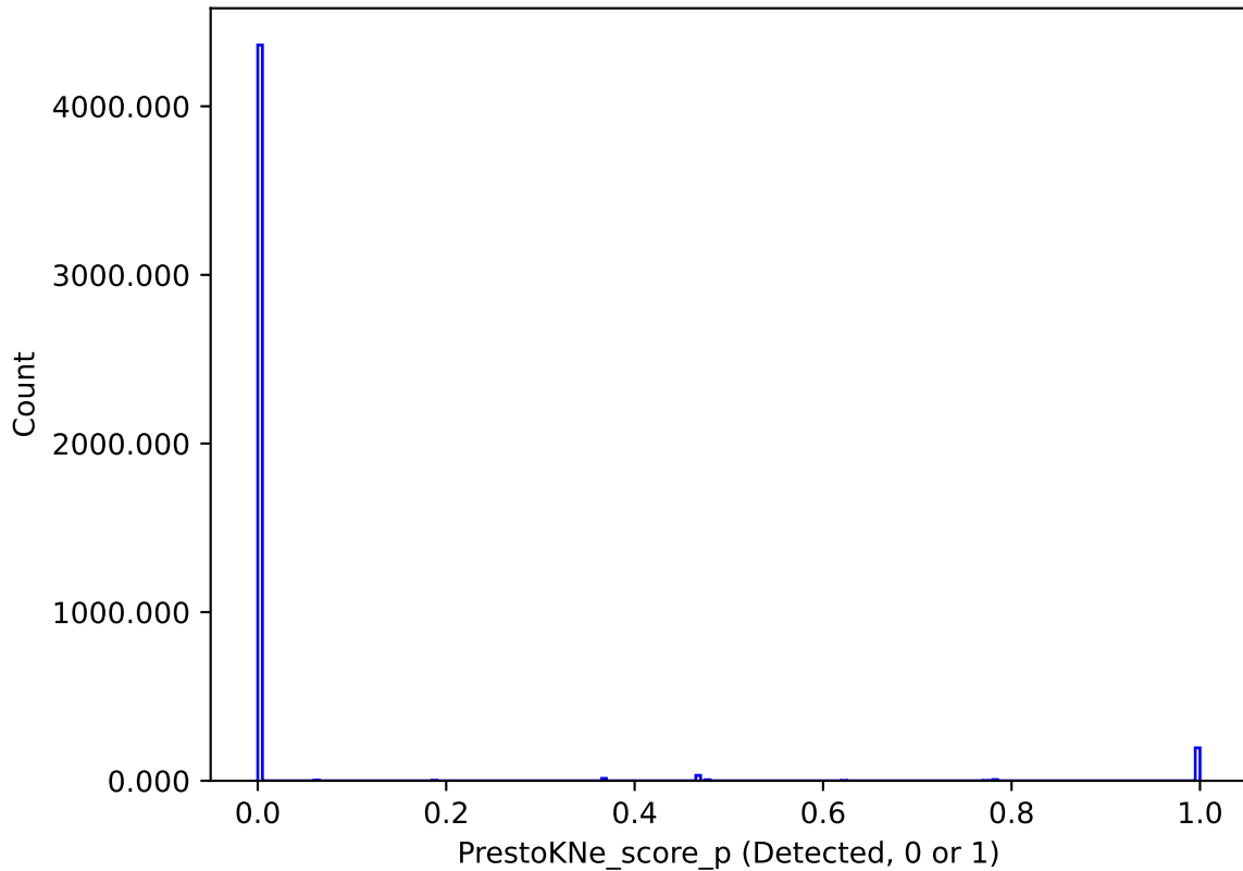
all_long_v3.4_10yrs : PrestoKNe_score_p
