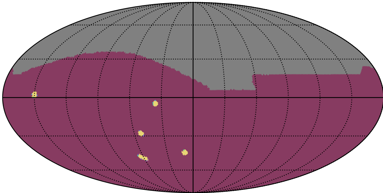
all_long_v3.4_10yrs : NumberOfQuickRevisits
