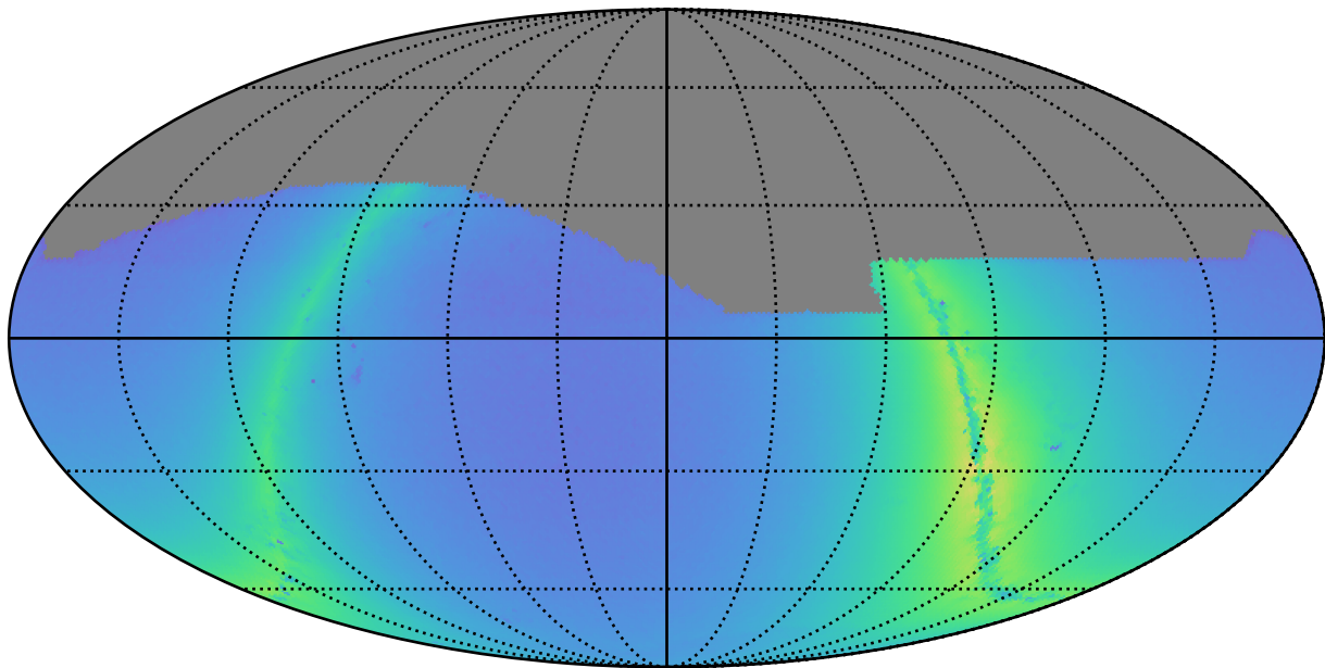
all_long_v3.4_10yrs z: Nstars_no_crowding
