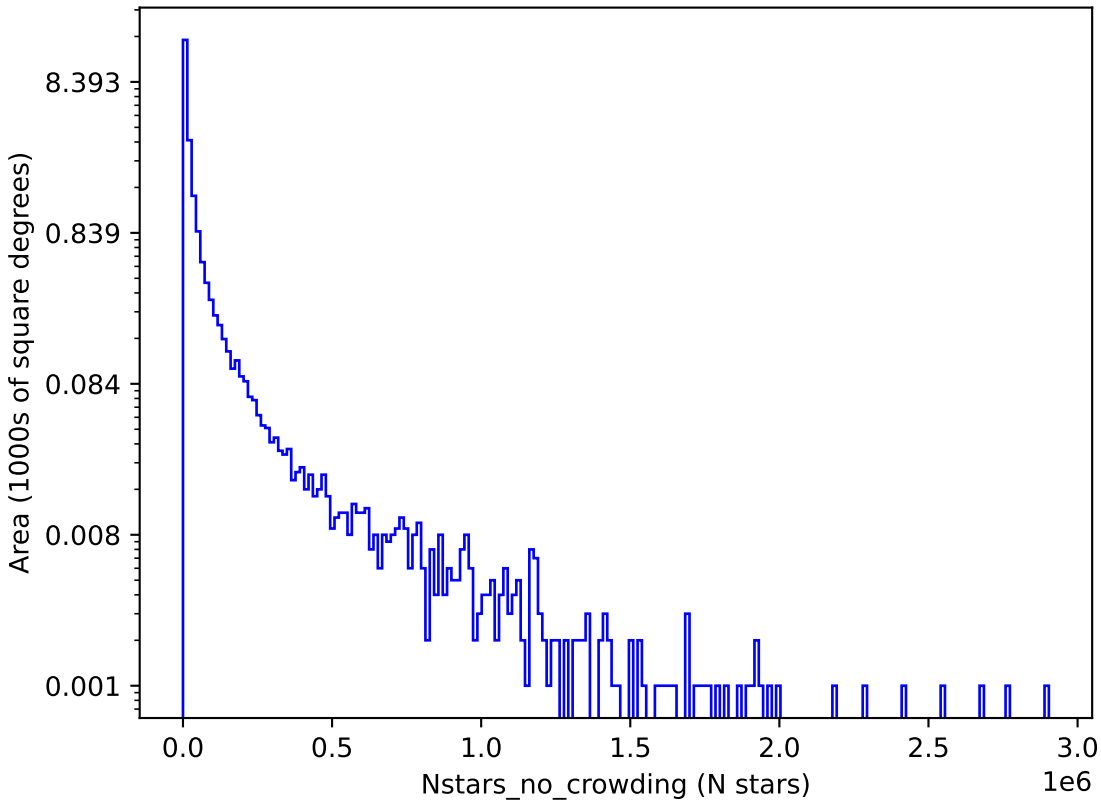
all_long_v3.4_10yrs u: Nstars_no_crowding
