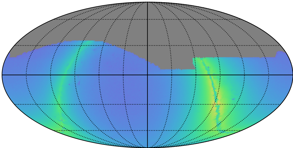
all_long_v3.4_10yrs i: Nstars_no_crowding
