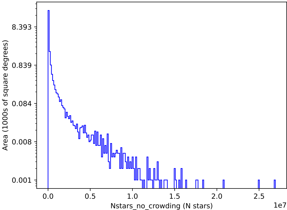
all_long_v3.4_10yrs i: Nstars_no_crowding
