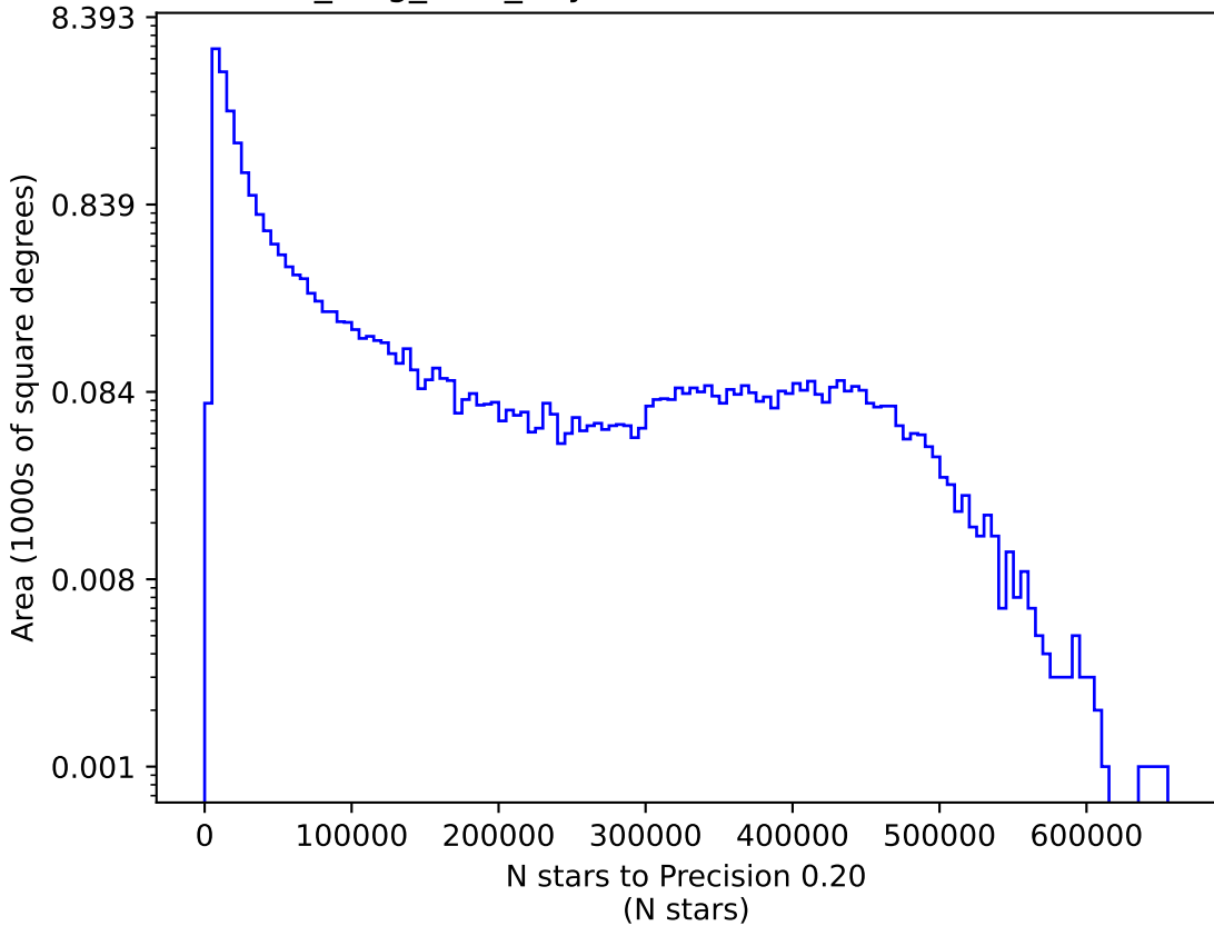
all_long_v3.4_10yrs i: N stars to Precision 0.20
