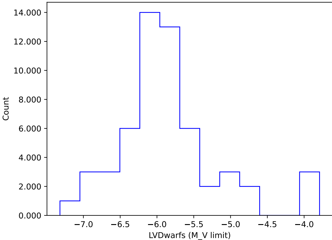
all_long_v3.4_10yrs gi: LVDwarfs
