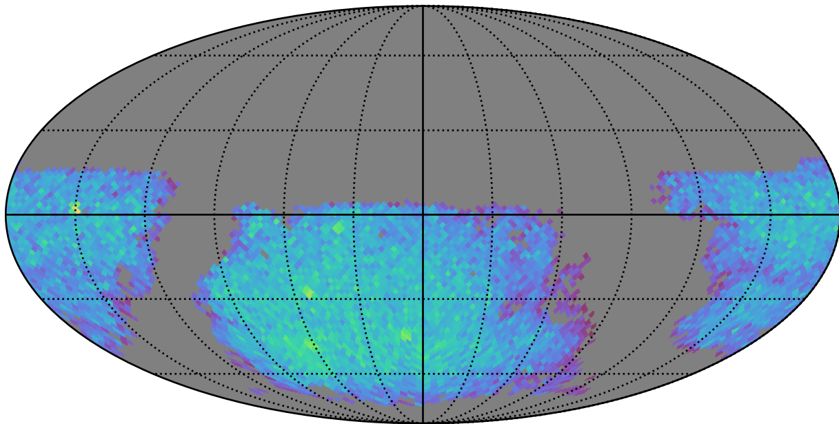
all_long_v3.4_10yrs gi: LVDwarfs
