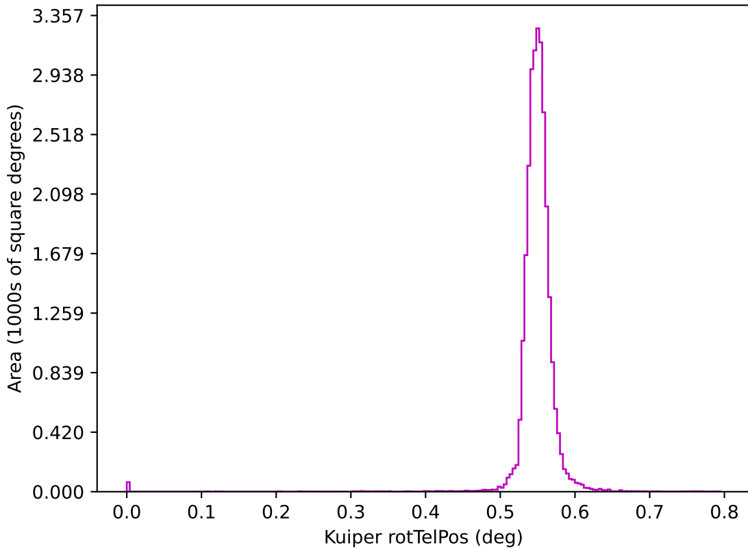
all_long_v3.4_10yrs z: Kuiper rotTelPos
