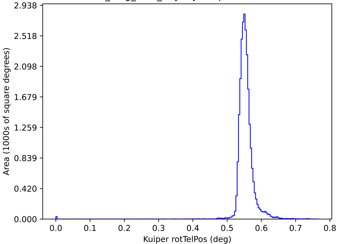
all_long_v3.4_10yrs y: Kuiper rotTelPos
