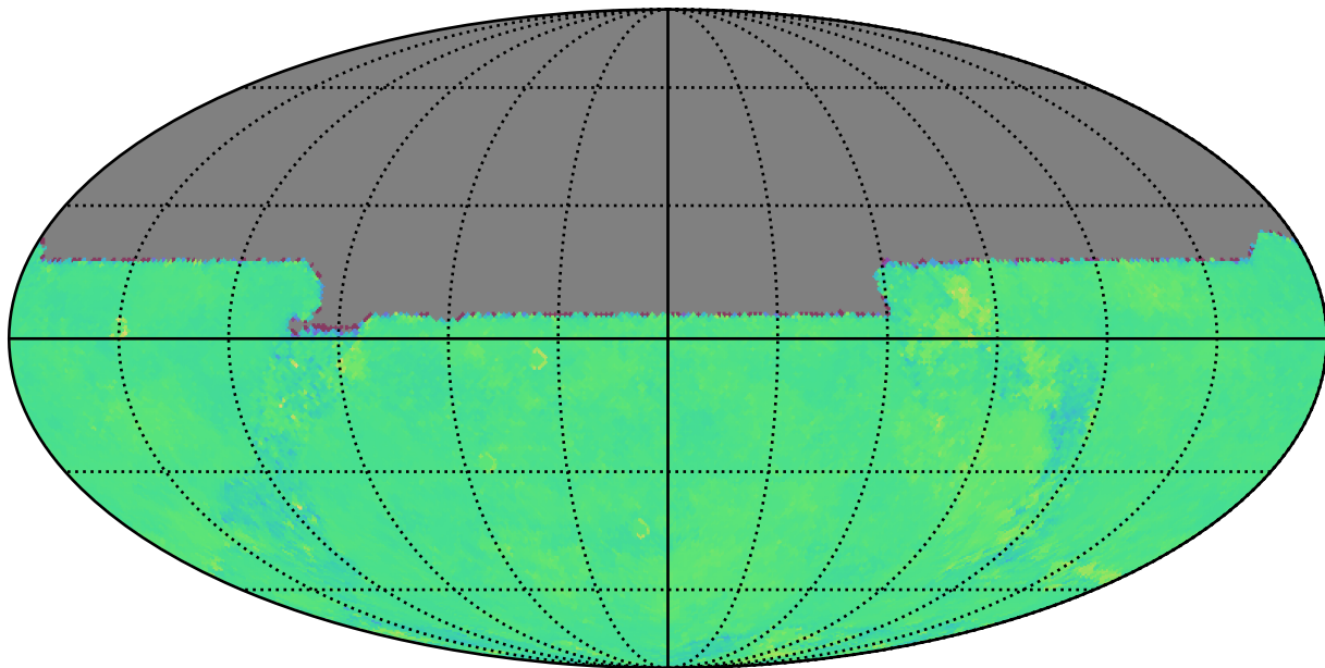
all_long_v3.4_10yrs u: Kuiper rotTelPos
