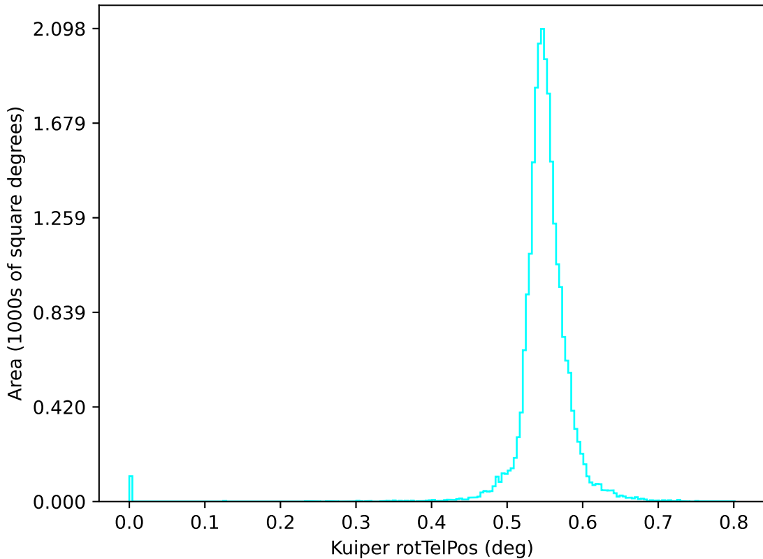
all_long_v3.4_10yrs u: Kuiper rotTelPos
