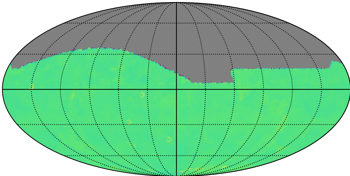
all_long_v3.4_10yrs r: Kuiper rotTelPos
