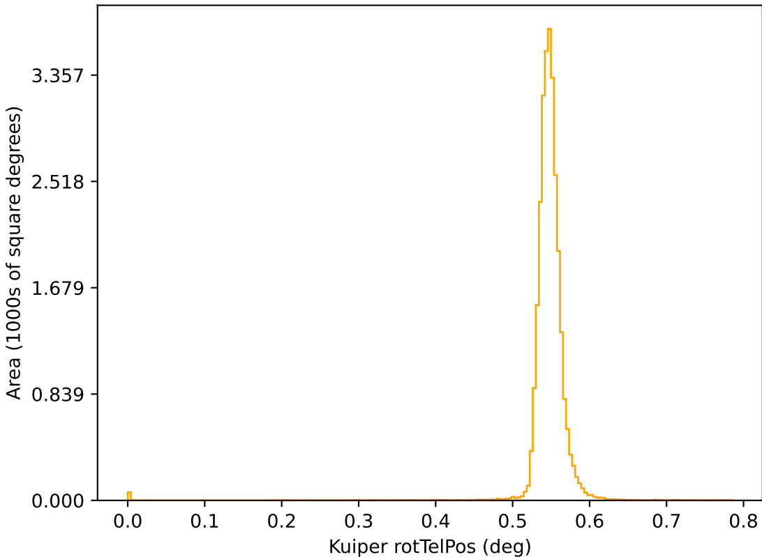
all_long_v3.4_10yrs r: Kuiper rotTelPos
