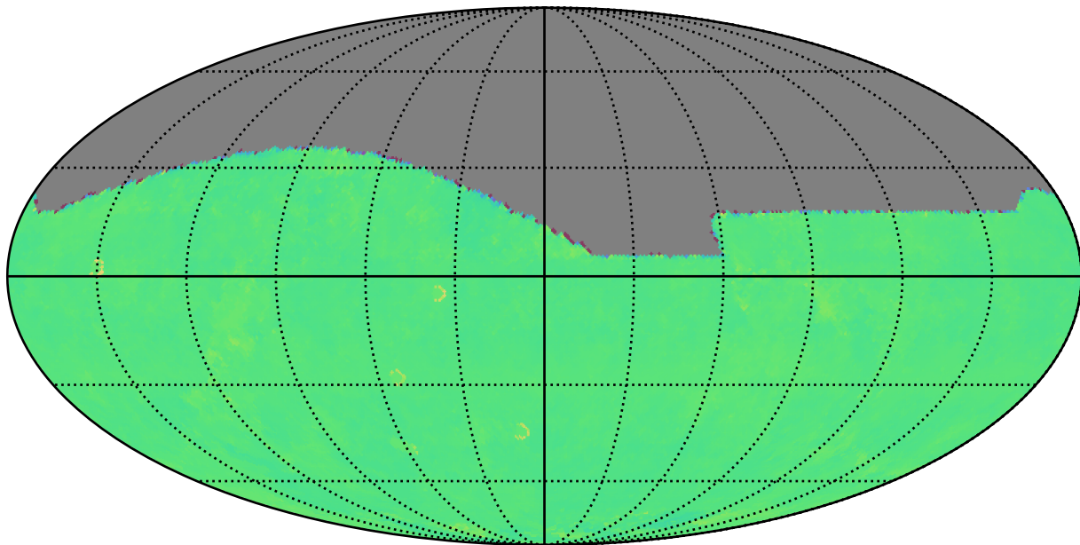
all_long_v3.4_10yrs i: Kuiper rotTelPos
