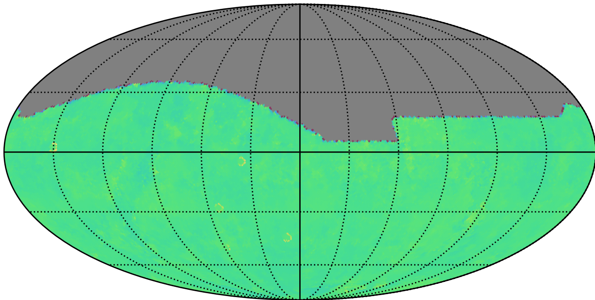
all_long_v3.4_10yrs g: Kuiper rotTelPos
