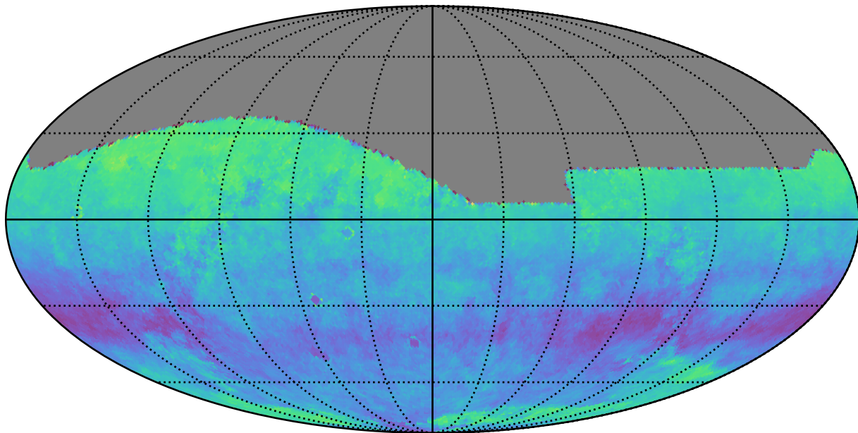
all_long_v3.4_10yrs z: Kuiper rotSkyPos
