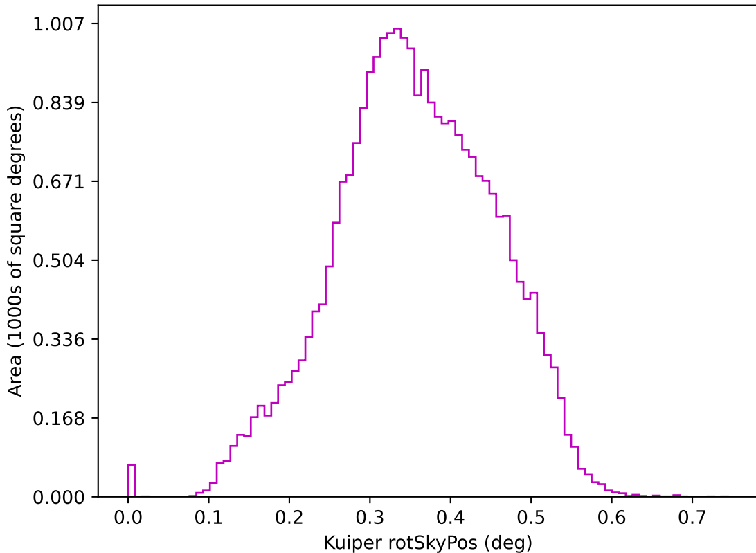
all_long_v3.4_10yrs z: Kuiper rotSkyPos
