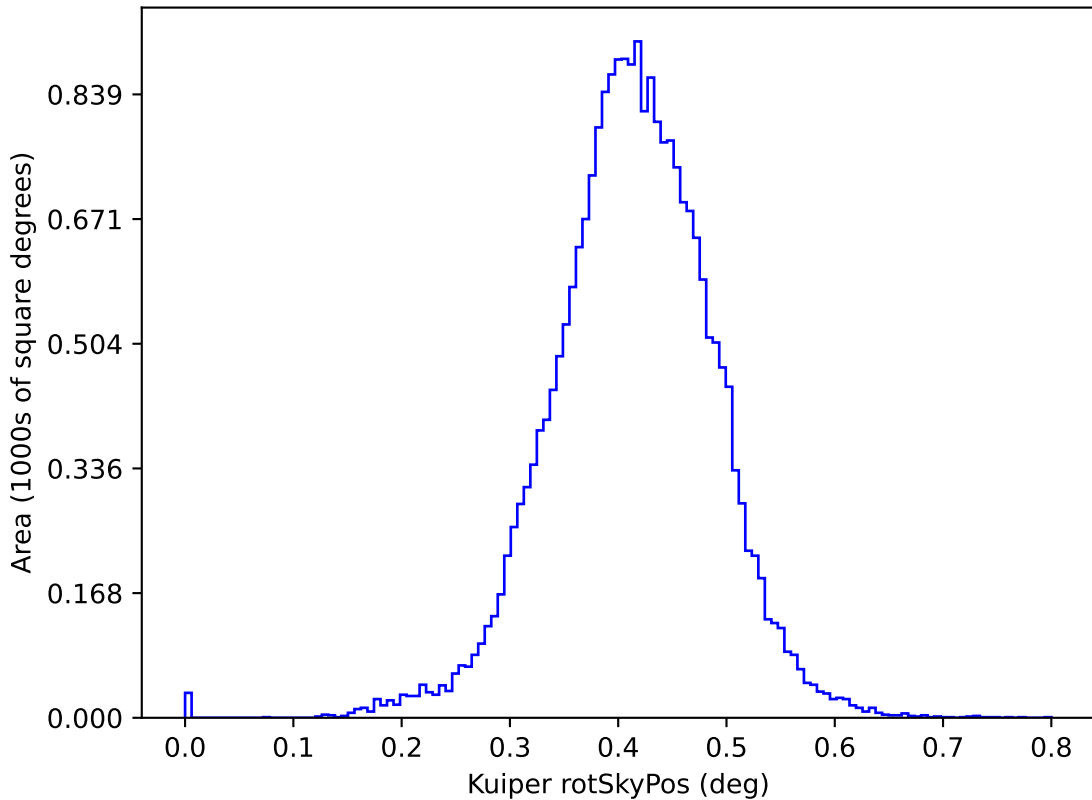
all_long_v3.4_10yrs y: Kuiper rotSkyPos
